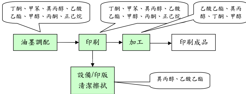
圖 4-2 塑膠印刷製造流程圖及可能暴露有害物的作業及有害物種類參考例
