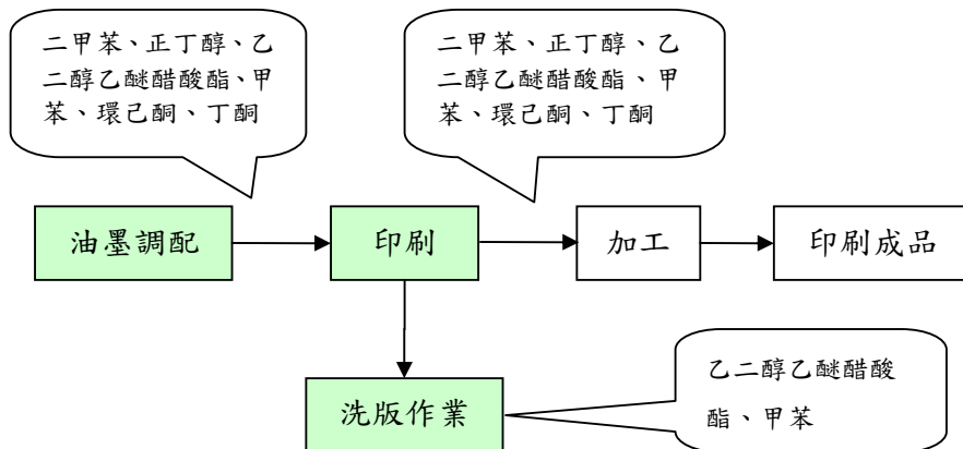
圖 4-3 網版印刷製造流程圖及可能暴露有害物的作業及有害物種類參考例
